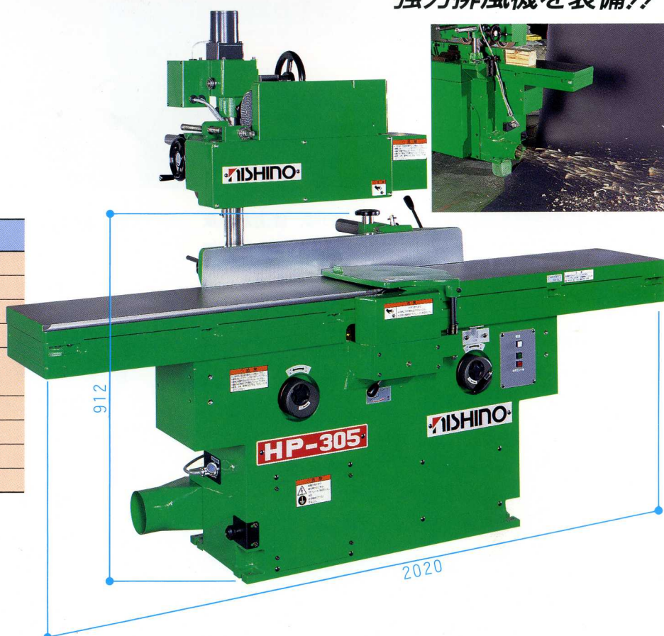
強力排風機装備(標準)
